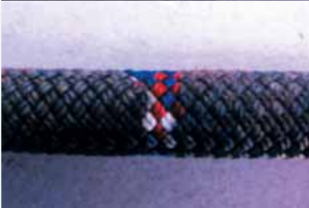
Abb. 14: Ausbleichen des Mantelgewebes; an der bunten Stelle war das Seil im Freien aufgehängt
