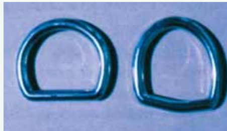
Abb. 18: Verformte Halteöse (rechts) nach Sturzbe- lastung oder miss- bräuchlicher Verwen- dung
